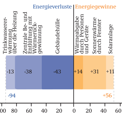
Ermittlung der Primärenergiebilanz dieses KfW-Energiesparhauses 40 (überschlägige Ermittlung)
