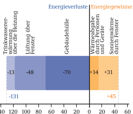
Ermittlung der Primärenergiebilanz dieses EnEV-Standard-Hauses (überschlägige Ermittlung)
